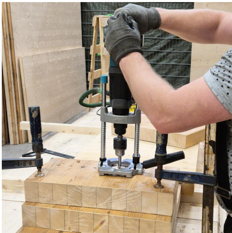
Closing loops- varastorakennus, liimapuiden työstö, Spolia Design
