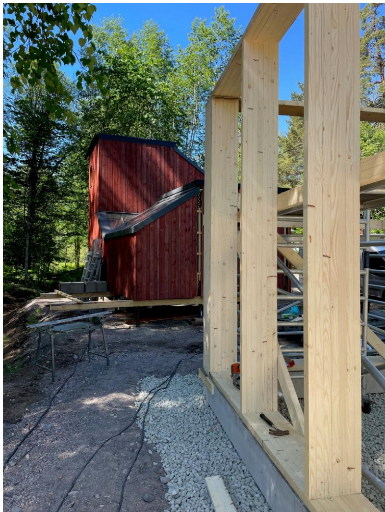
Autotalli, Fiskars. Kuvat: Johanna Hyrkäs
